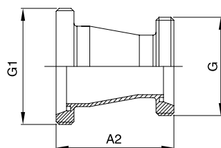
(螺纹式 Threaded)
