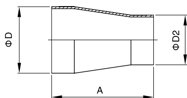
(同心 Concentric)
