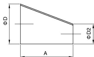
(偏心 Eccentric)
