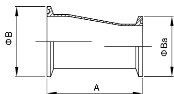
(偏心 Eccentric)
