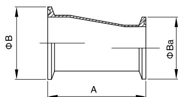
(偏心 Eccentric)
