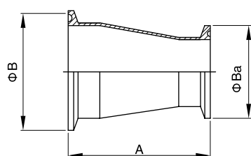
(同心 Concentric)
