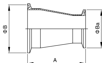
(同心 Concentric)
