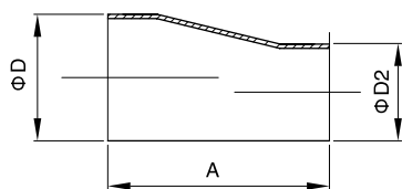
(偏心 Eccentric)
